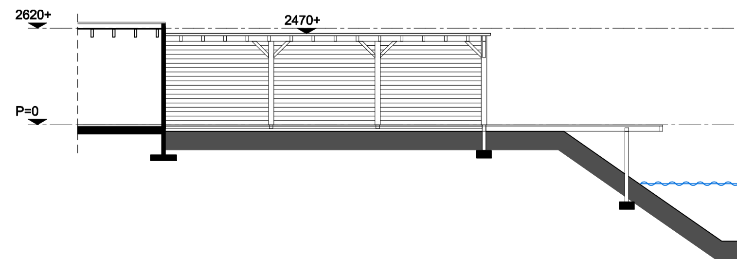
doorsnede
