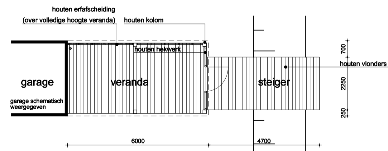
begane grond
