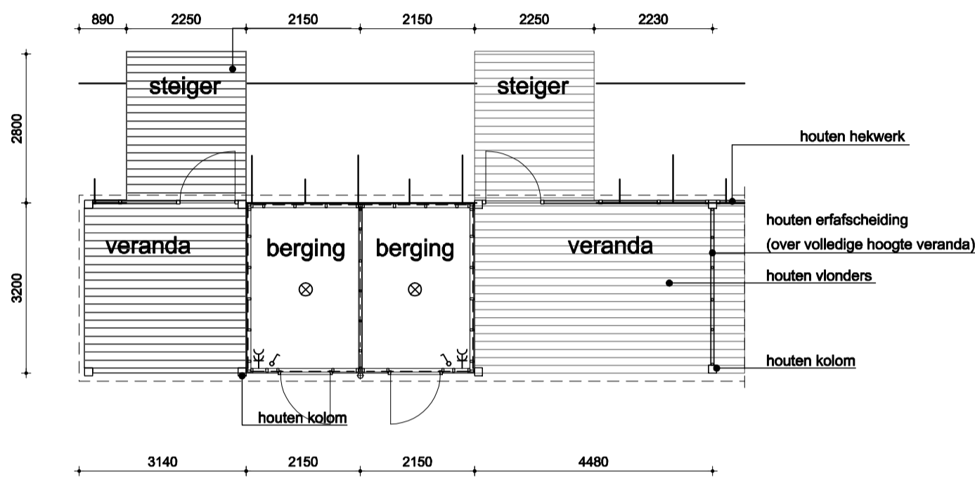
begane grond
