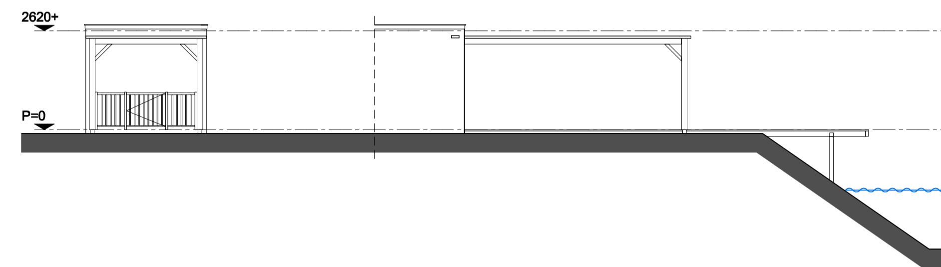
achtergevel
