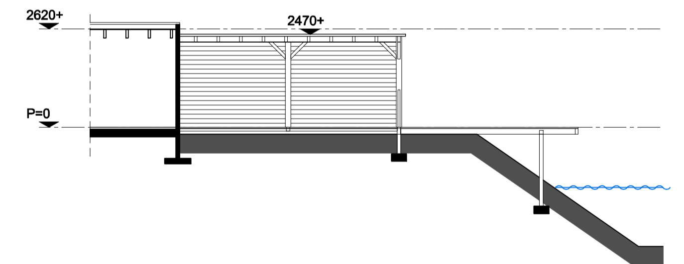
doorsnede
