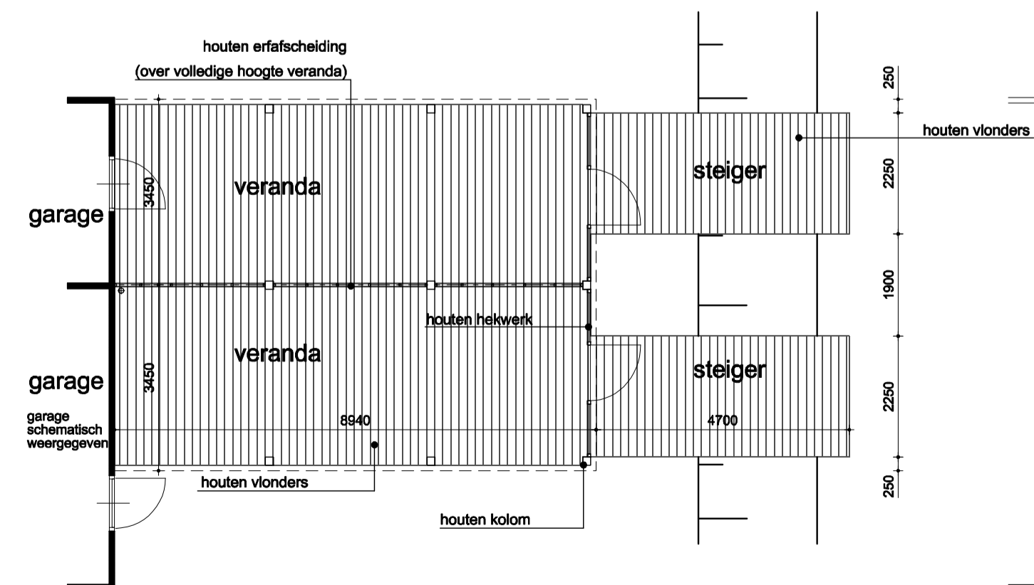
begane grond
