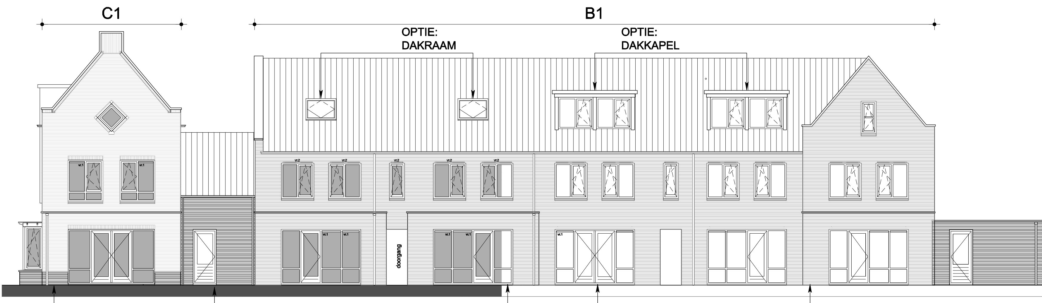
VOORGEVEL, schaal 1:100
