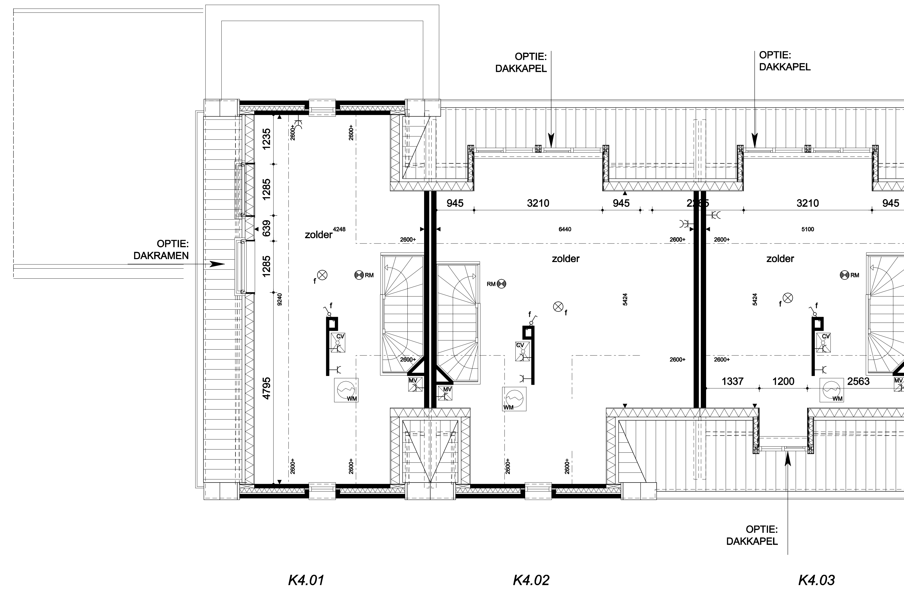
ZOLDER, schaal 1:50
