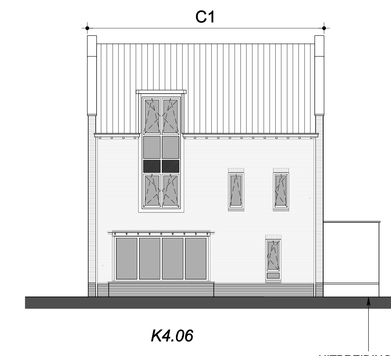
RECHTER ZIJGEVEL, schaal 1:100
