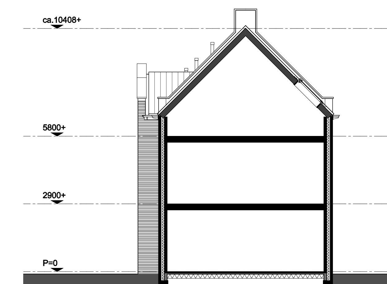
DOORSNEDE, schaal 1:100
