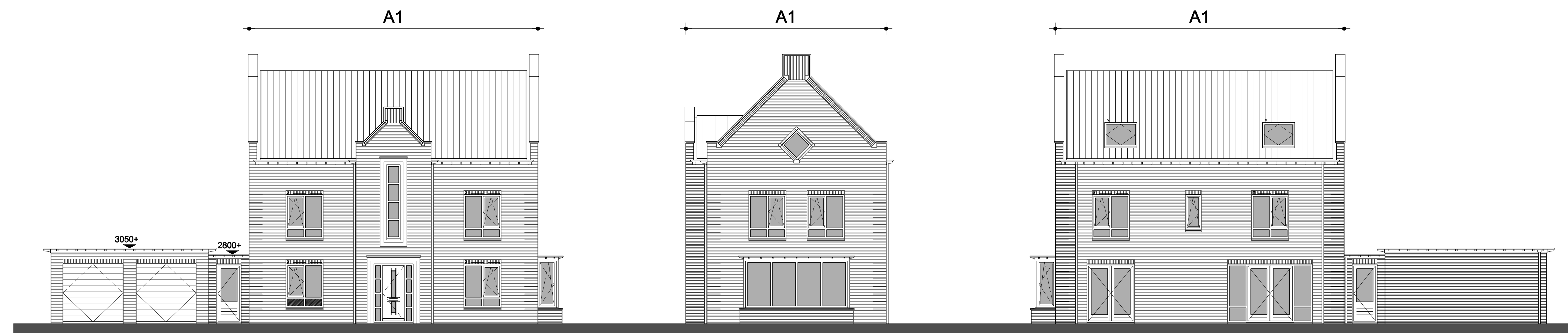
VOORGEVEL, schaal 1:100
