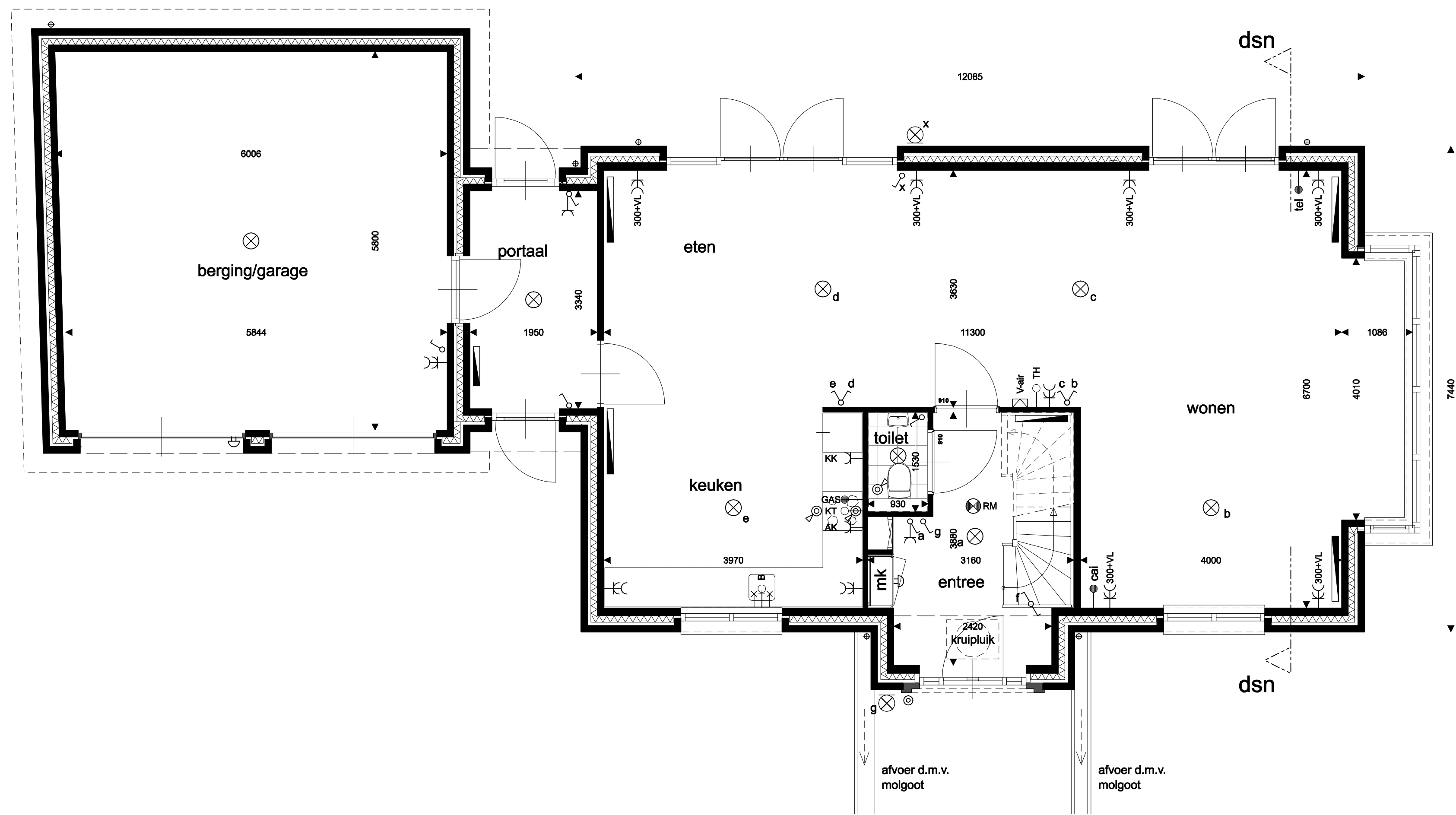
BEGANE GROND, schaal 1:50
