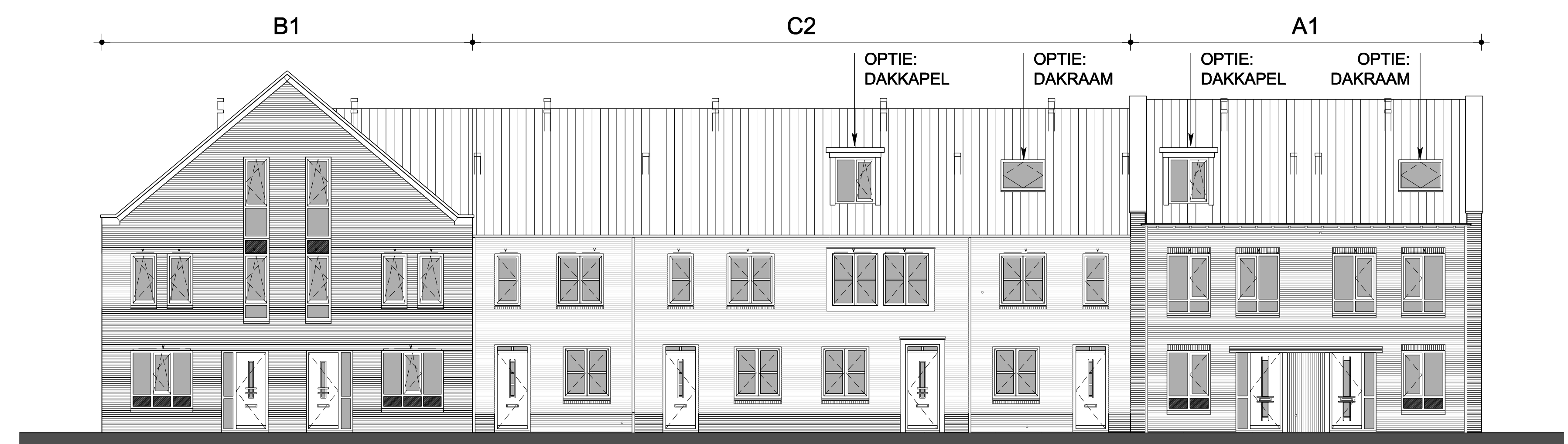
VOORGEVEL, schaal 1:100
