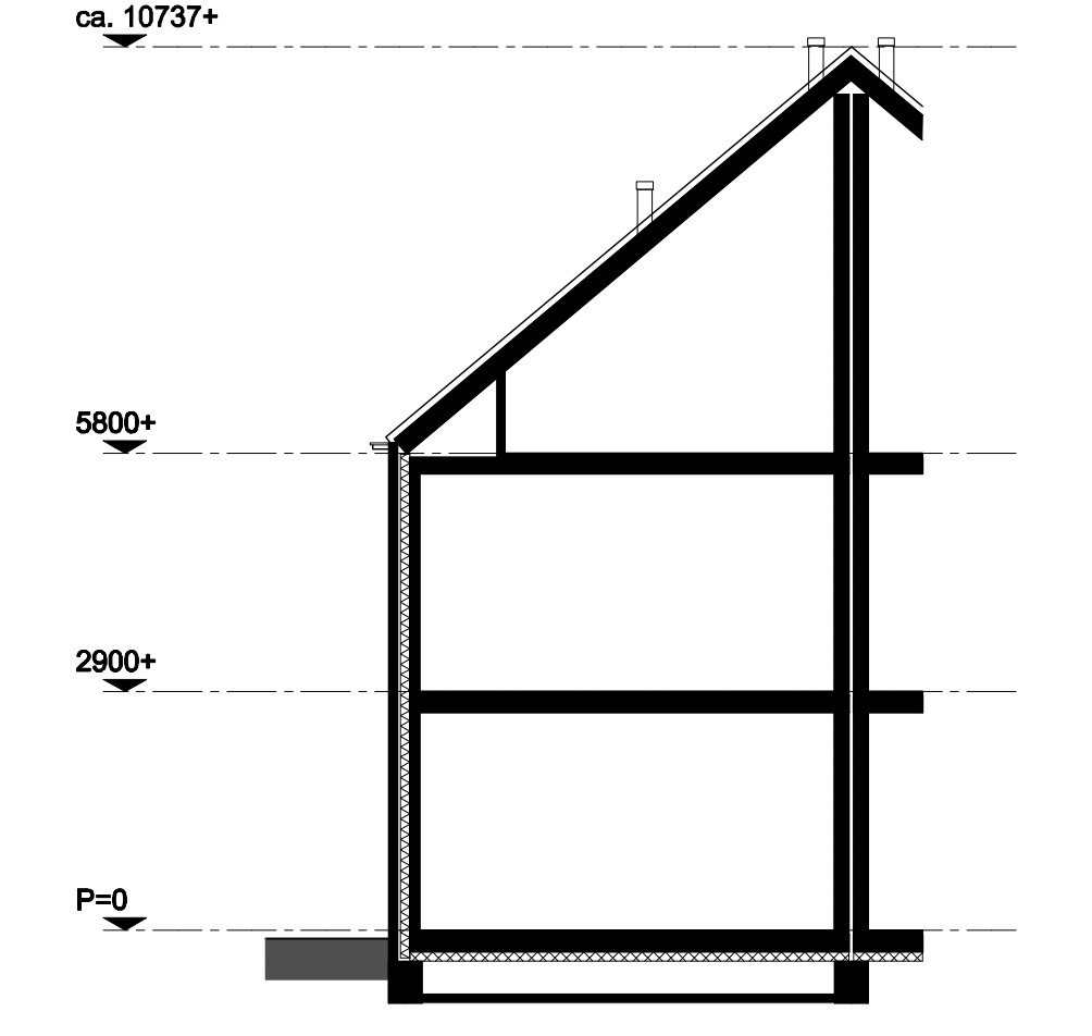
DOORSNEDE, schaal 1:100
