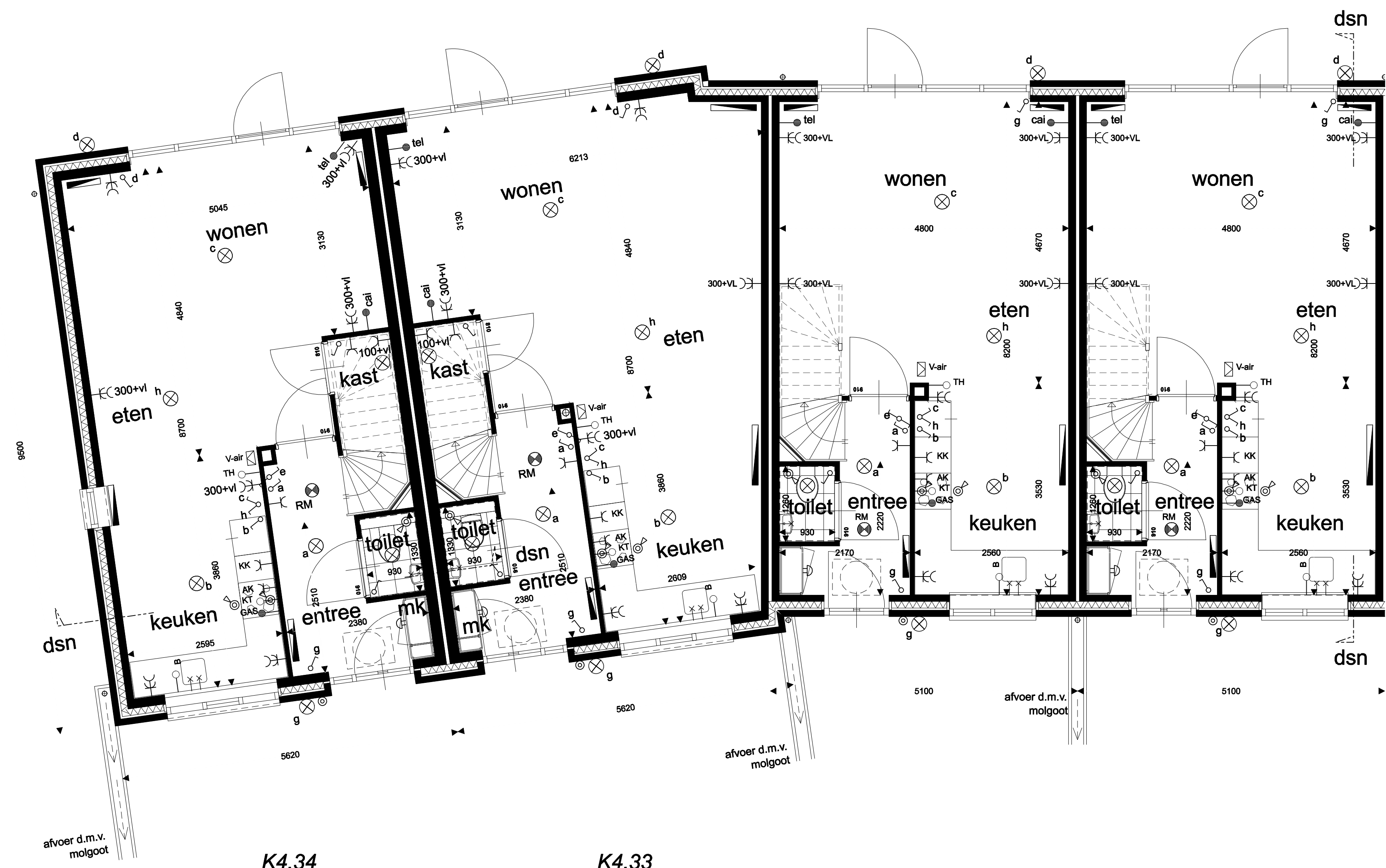
BEGANE GROND, schaal 1:50
